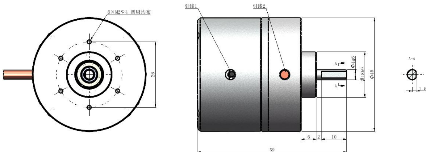
R45-S 外形尺寸图
