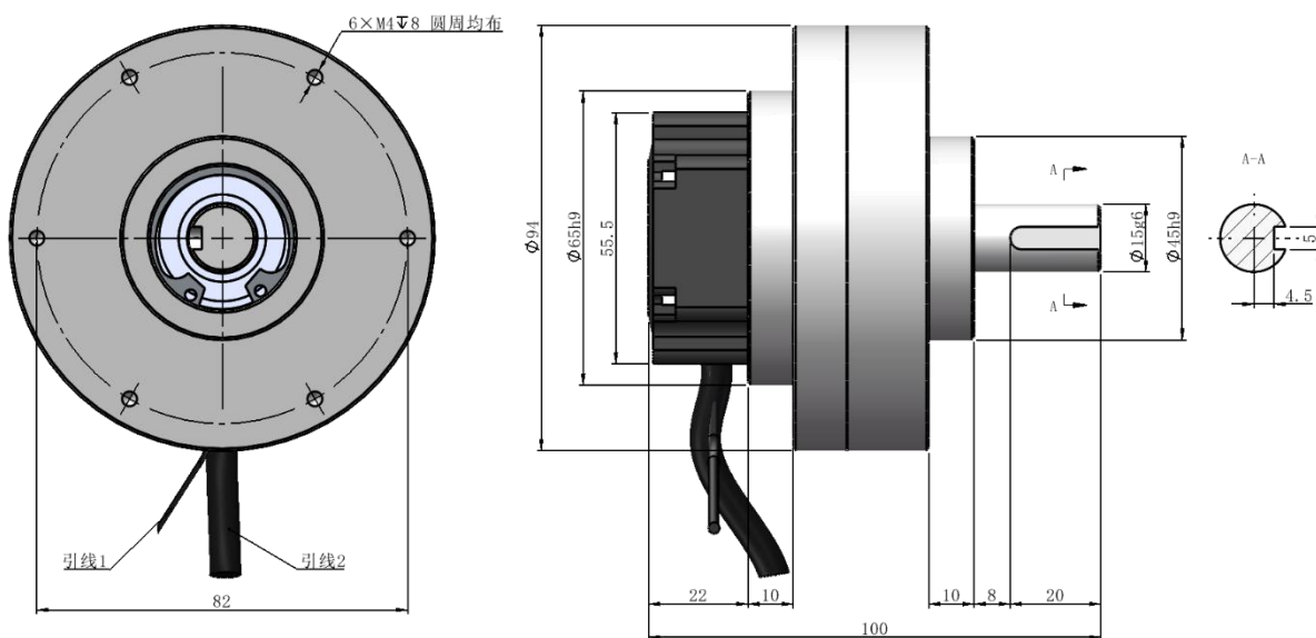
R94-S 外形尺寸图
