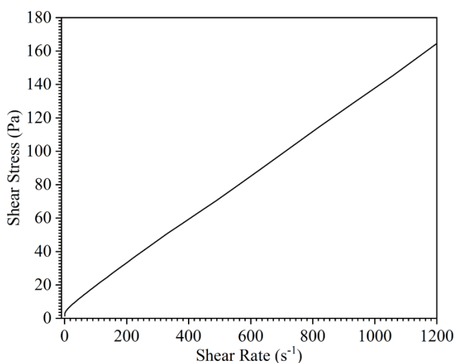
Fig 1: 40°C零磁场下剪切应力与剪切速率关系
