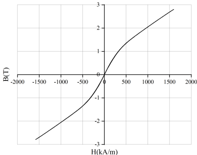
Fig 4: 磁感应强度与磁场强度关系
